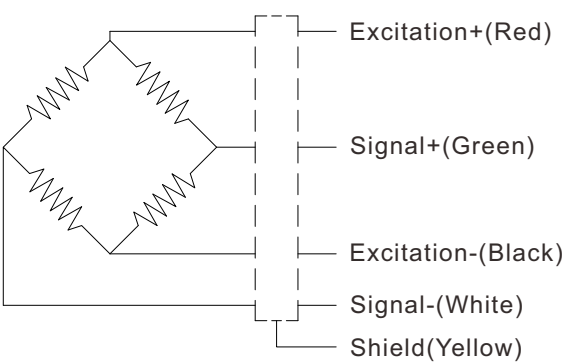
Wiring Code@Clockwise
