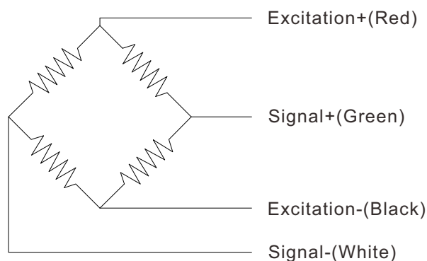
Wiring Code
